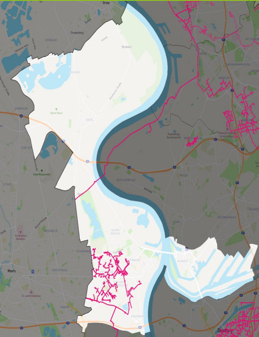
Derzeitiges Wärmenetz im Bezirk Homberg, Ruhrort, Baerl
